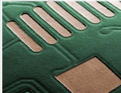
Lötstopplack öffnen, Taschen und blind vias erzeugen
